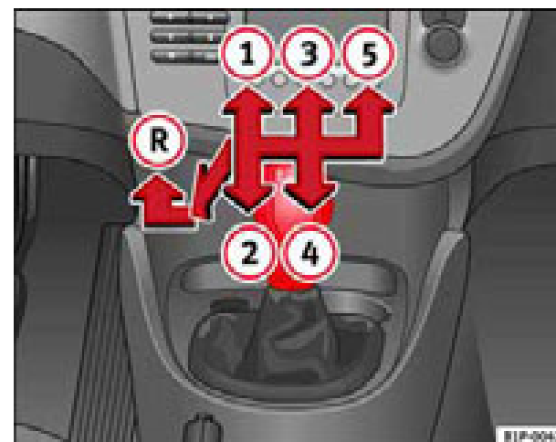
Fig. 114 Detalle de la consola central: esquema de un cambio manual de 5 marchas
