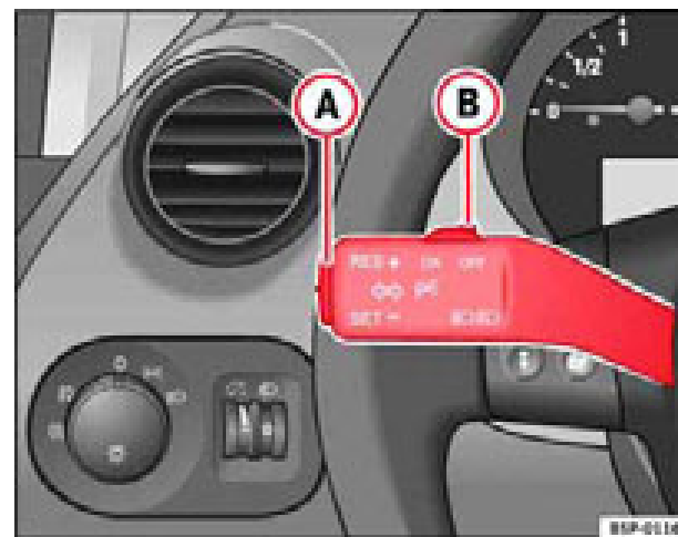
Fig. 126 Palanca de intermitentes y de luz de carretera: mando y tecla basculante para el regulador de velocidad
