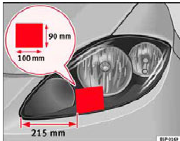
Fig. 128 Faro izquierdo
