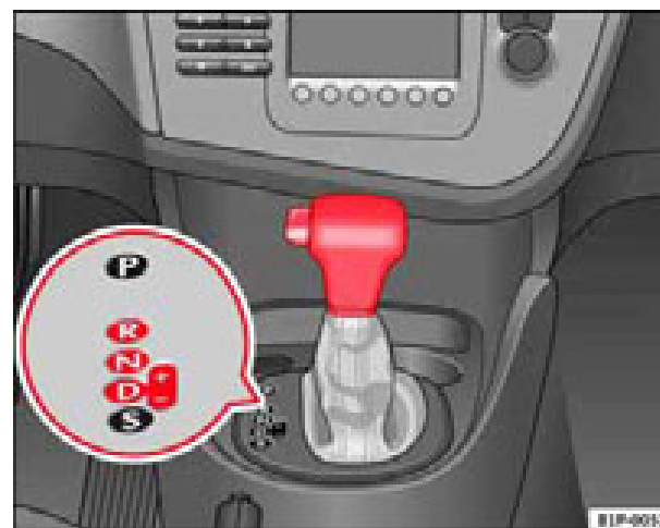
Fig. 118 Desactivación del bloqueo
