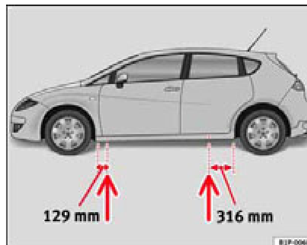
Fig. 149 Puntos de apoyo del gato
