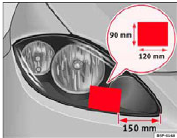
Fig. 127 Faro derecho
