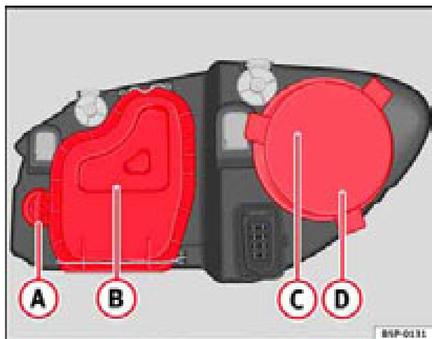
Fig. 155 Lámparas del faro principal
