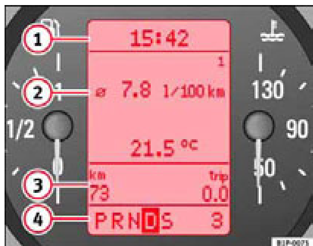
Fig. 37 Pantalla digital del cuadro de instrumentos
