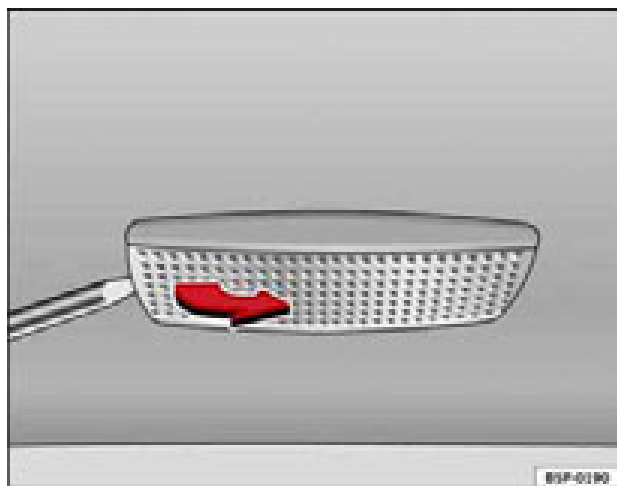
Fig. 171 Desmontaje luz del parasol
