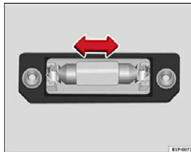
Fig. 170 Luz matrícula
