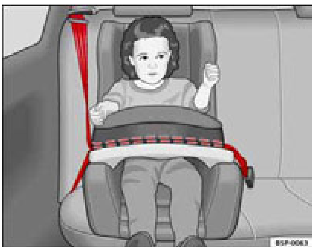
Fig. 28 Asiento para niños del grupo 1 montado en el asiento trasero en la dirección de la marcha.
