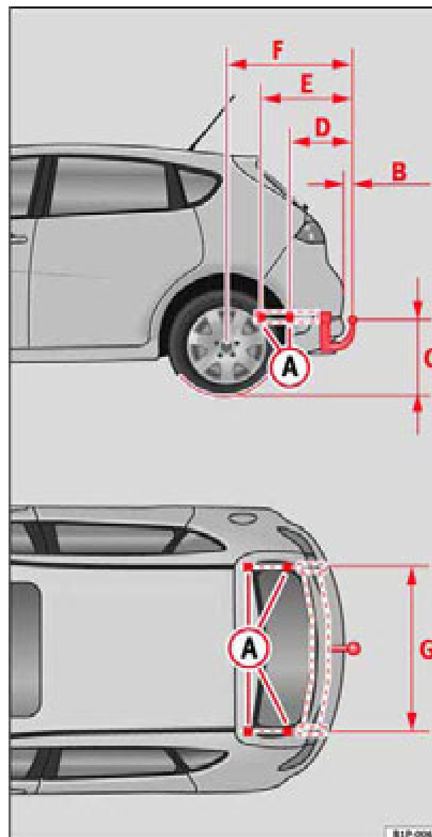
Fig. 132 Puntos de fijación del dispositivo de remolque
