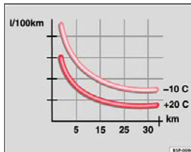
Fig. 131 Consumo de combustible (l/100 km) a dos temperaturas ambiente
