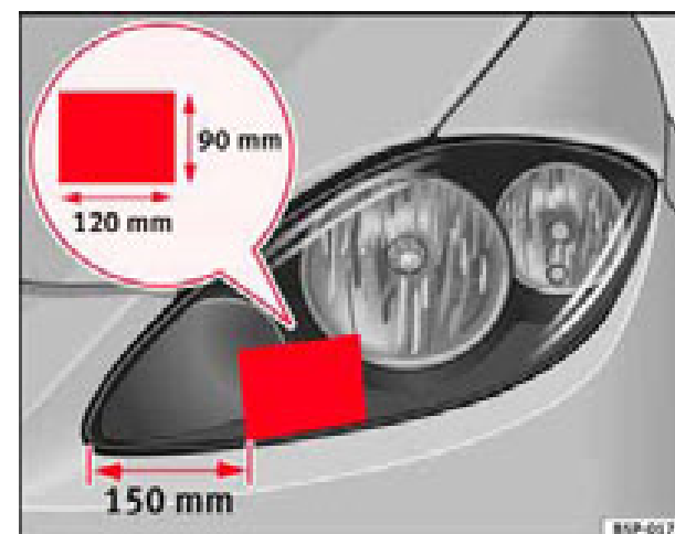
Fig. 130 Faro izquierdo ►
