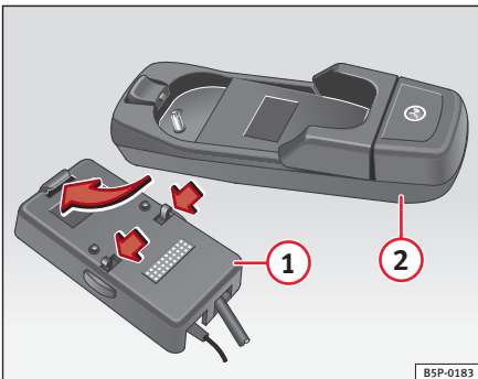
Fig. 3 Montaje del adaptador
